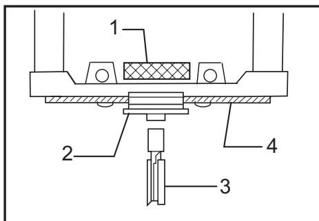
► 1. Contratuera 2. Guía de plantilla 3. Broca del router 4. Placa base
